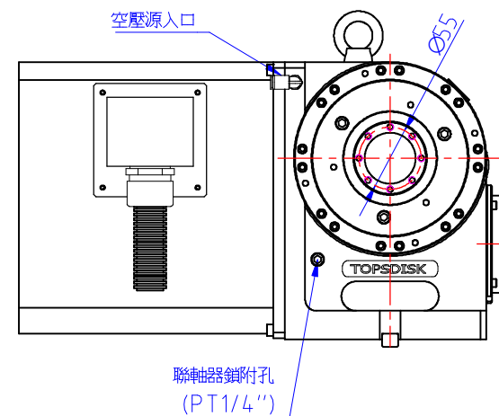
主軸尺寸示意圖
