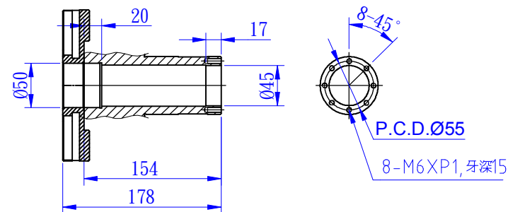
主軸尺寸示意圖
