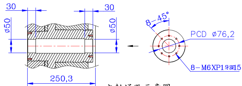
主軸通孔示意圖
