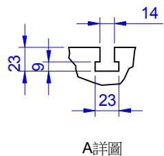
A詳圖
