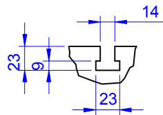
A詳圖
