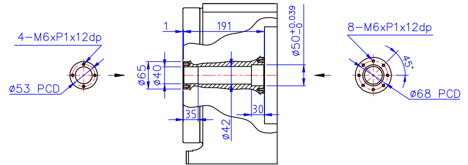
A-A主軸剖視示意圖
