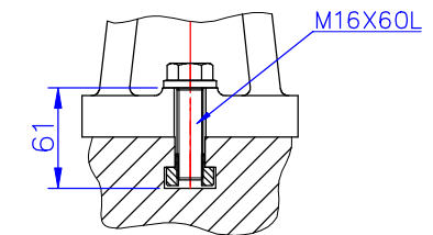
與18T溝配合螺絲長度示意圖
