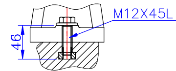
與14T溝配合螺絲長度示意圖
