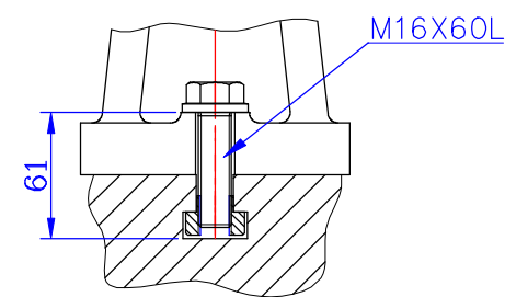
與18T溝配合螺絲長度示意圖
