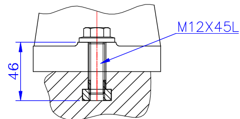
與14T溝配合螺絲長度示意圖
