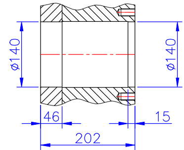
通孔尺寸示意圖
