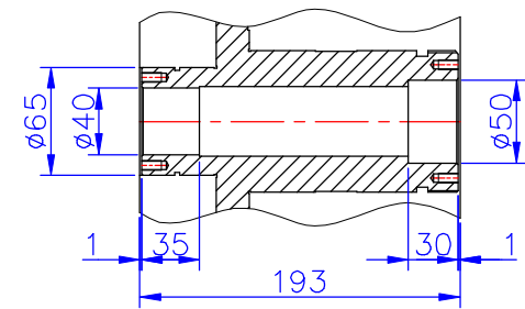
主軸通孔尺寸示意圖
