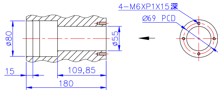
主軸通孔尺寸示意圖
