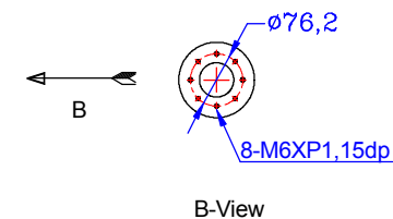
B-View
