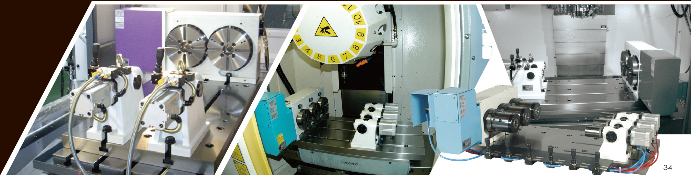
▼ 多主軸NC旋轉工作台應用 Multi-spindle NC Rotary Table
